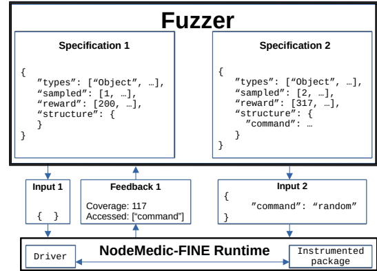
Fig. 4: Fuzzer loop
